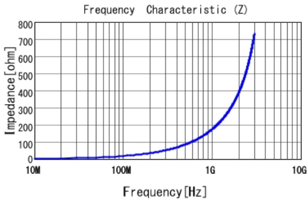
LQW04AN27NH00 |Z|
