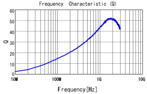
LQW04AN27NH00 Q
