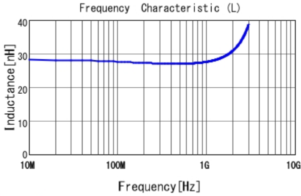
LQW04AN27NH00 L
