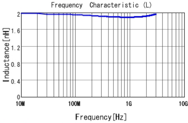
LQW04AN1N9C00 L
