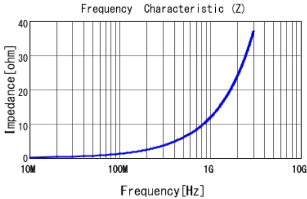
LQW04AN1N9C00 |Z|
