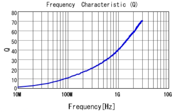
LQW04AN1N9C00 Q
