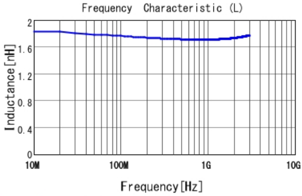
LQW04AN1N7D00 L
