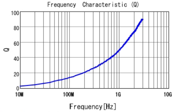
LQW04AN1N7D00 Q
