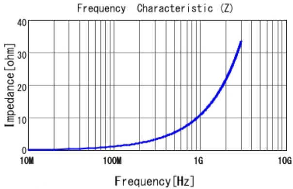
LQW04AN1N7D00 |Z|
