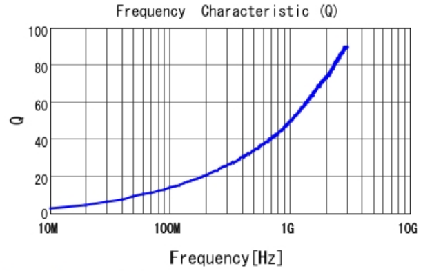
LQW04AN1N7C00 Q
