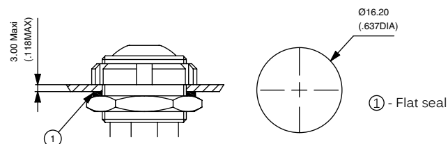
IZM (adjustable hex nut)
