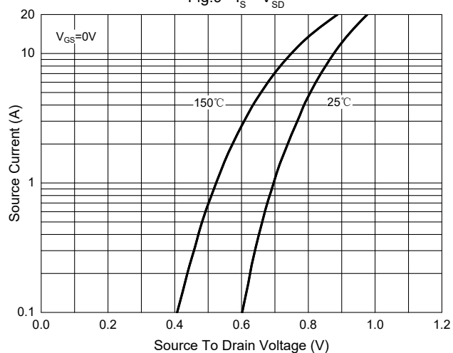
Fig.9 - I_S - V_{SD}
