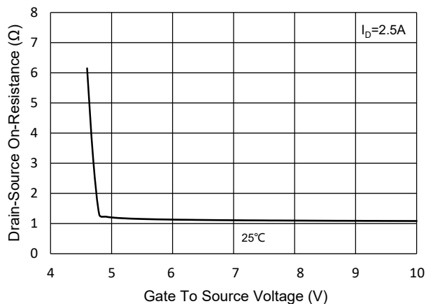
Fig.3 - R_{DS(ON)} - V_{GS}
