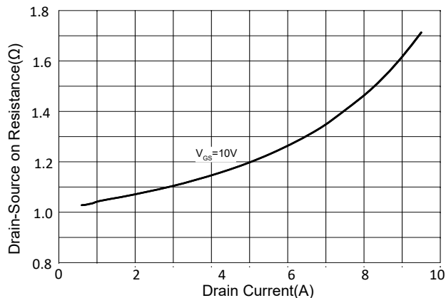
Fig. 4 - R_{DS(ON)} - I_D
