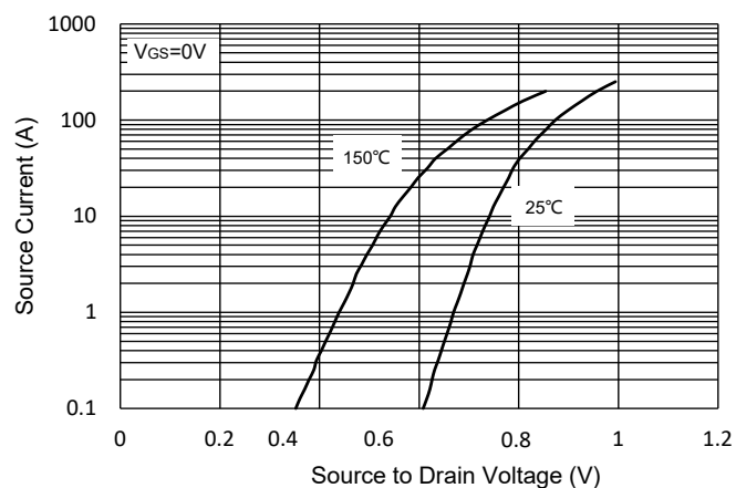
Fig.9 - I_S - V_{SD}
