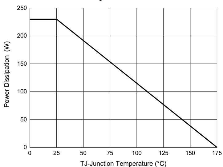
Fig. 11 - PD— T_J
