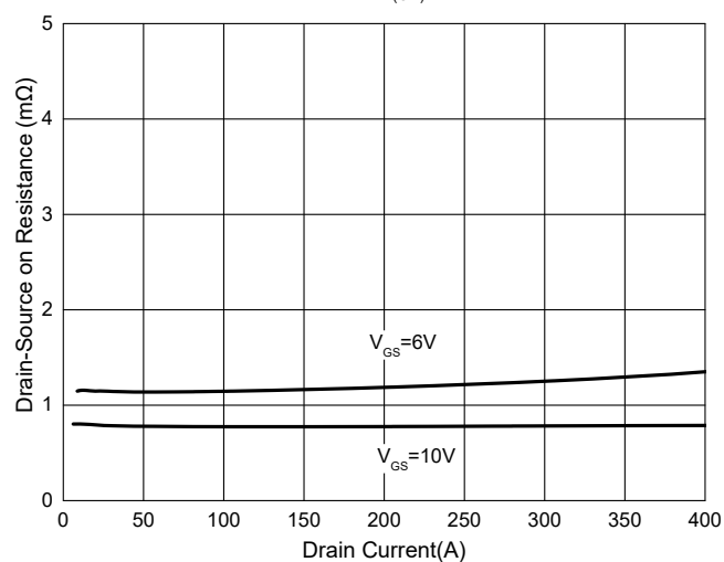
Fig. 7 - R_{DS(ON)} - I_D
