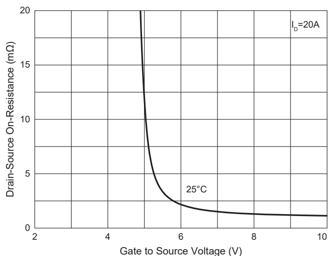
Fig. 3 - R_{DS(ON)} - V_{GS}
