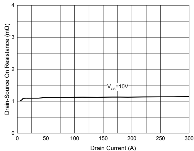
Fig. 4 - R_{DS(ON)} - I_D
