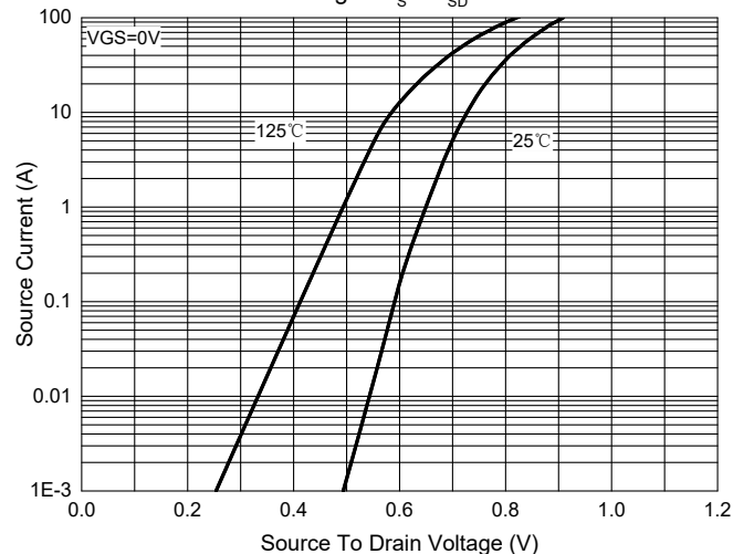
Fig.9 - I_S - V_{SD}
