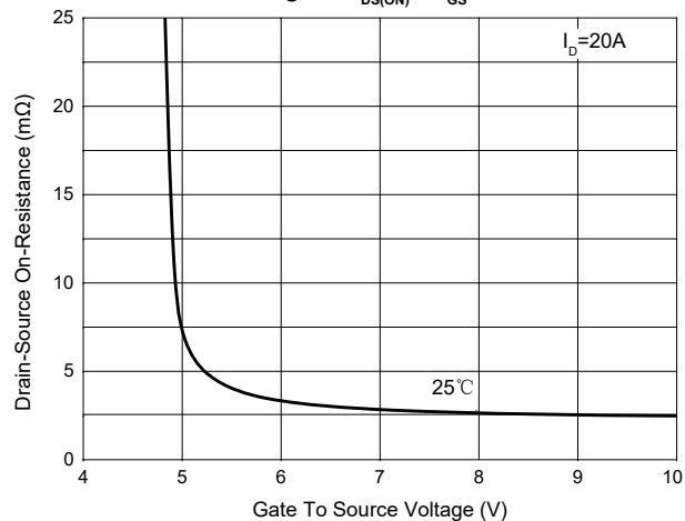
Fig. 3 - R_{DS(ON)} — V_{GS}
