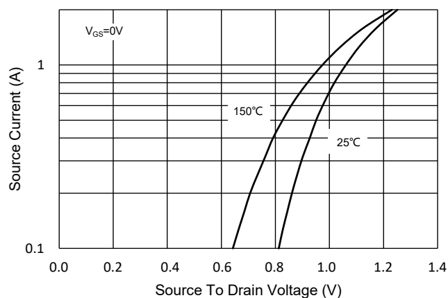
Fig.9 - I_S - V_{SD}
