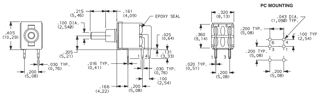
EP21SD1ABE DPST
