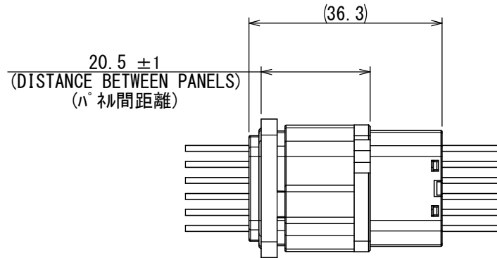
CONNECTOR MATING STATE コネクタ嵌合状態
