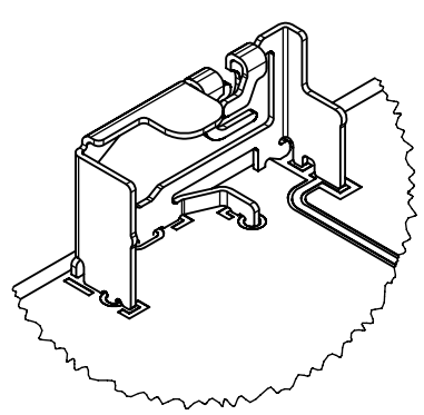
PERSPECTIVE VIEW 斜視図 SCALE 2:1
