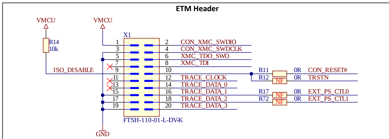
Figure 19 ETM header
