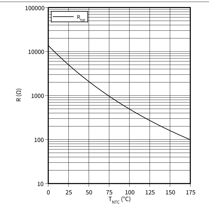
Temperaturkennlinie (typisch), NTC-Widerstand R = f(T_{NTC})
