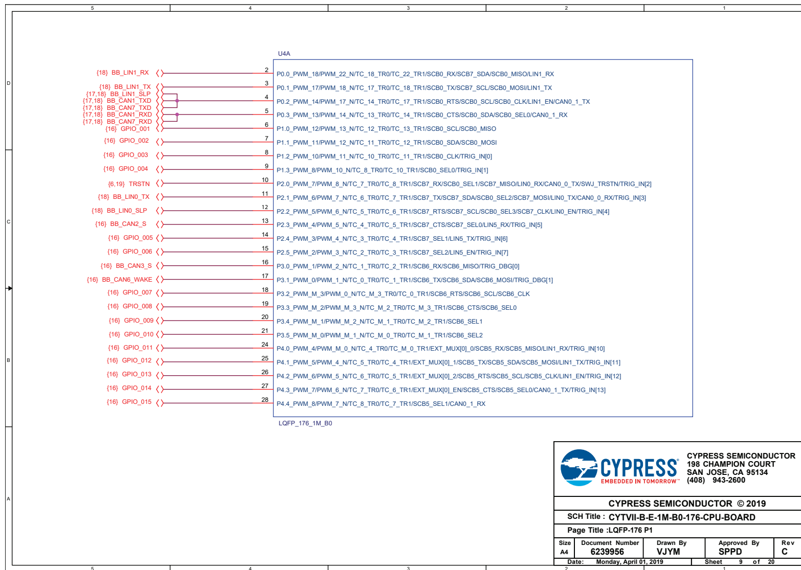
Figure A-8. LQFP-176 P1
