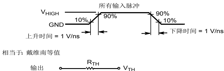
图 7. 交流测试负载和波形 [18]
