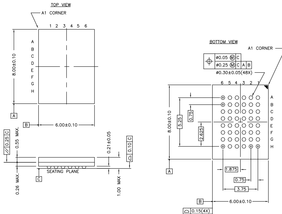
图 17. 48 球形焊盘 VFBGA (6 × 8 × 1.0 mm) BV48/BZ48 封装外形, 51-85150
