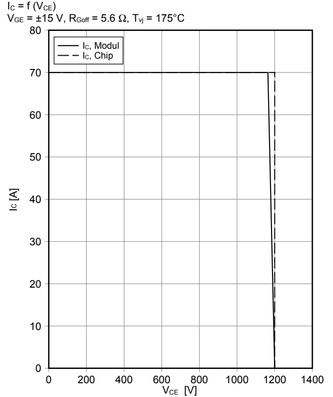
Sicherer Rückwärts-Arbeitsbereich IGBT, Wechselrichter (RBSOA) reverse bias safe operating area IGBT, Inverter (RBSOA) I_C = f(V_{CE}) V_{GE} = \pm 15\text{ V} , R_{Goff} = 5.6\ \Omega , T_{vj} = 175^\circ\text{C}
