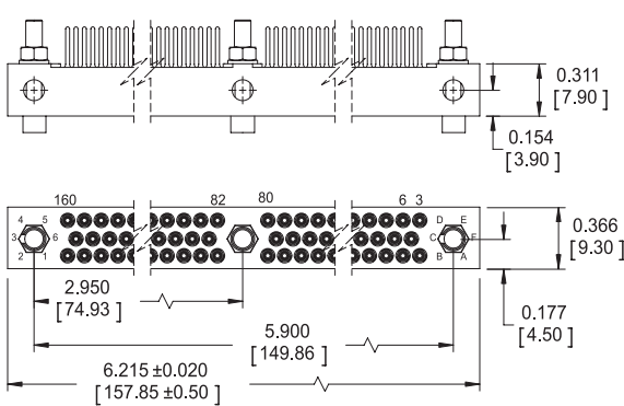
Receptacle
