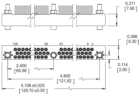
Receptacle
