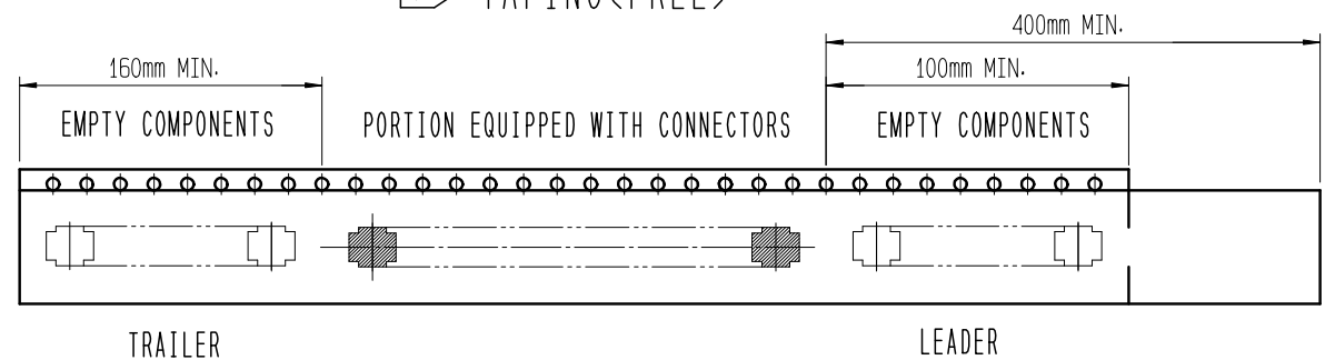
9 TAPING(FREE)
