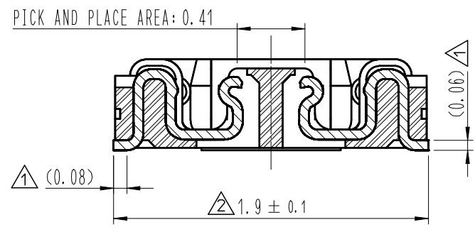
A-A (30:1)
