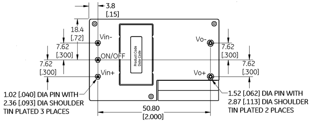
BOTTOM VIEW***
