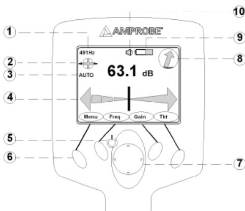
R-5000 Bedienungsfläche
