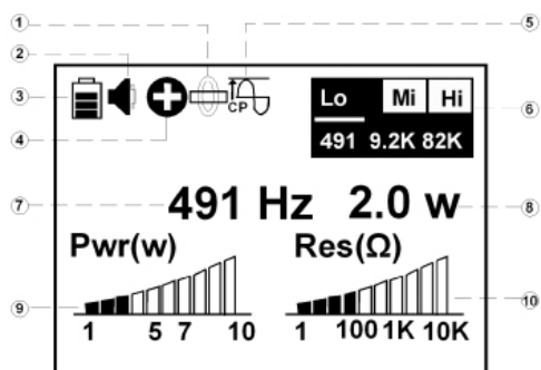
LCD till T-5000:s driftsgränssnitt
