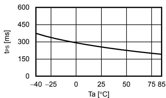
3. 12 t_{PS} vs. T_a
