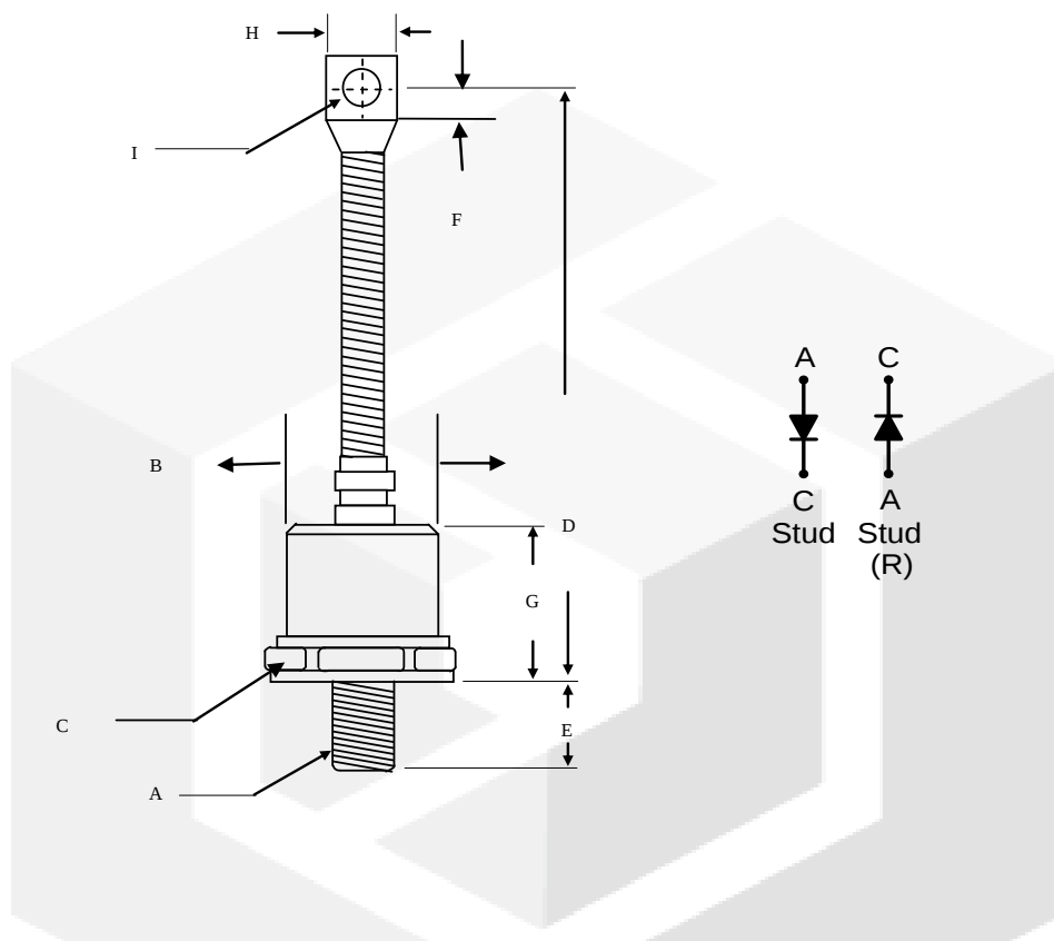
DO-9 (DO--205AB)
