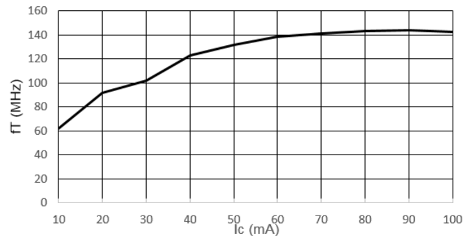
f_T vs I_C
