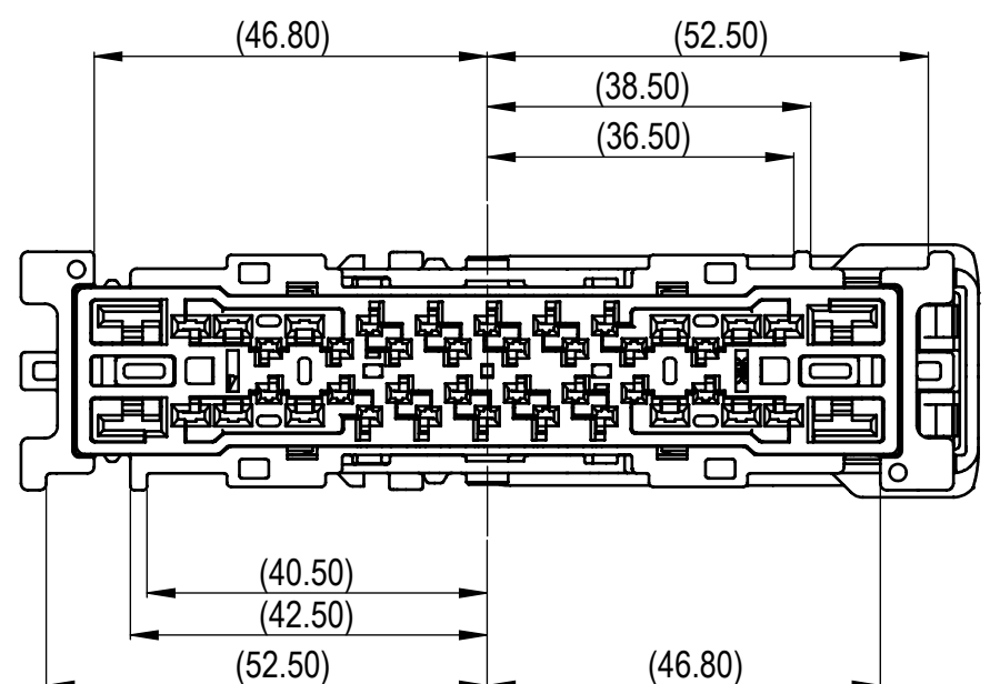
7287-8884-60 KEYWAY C RIGHT
