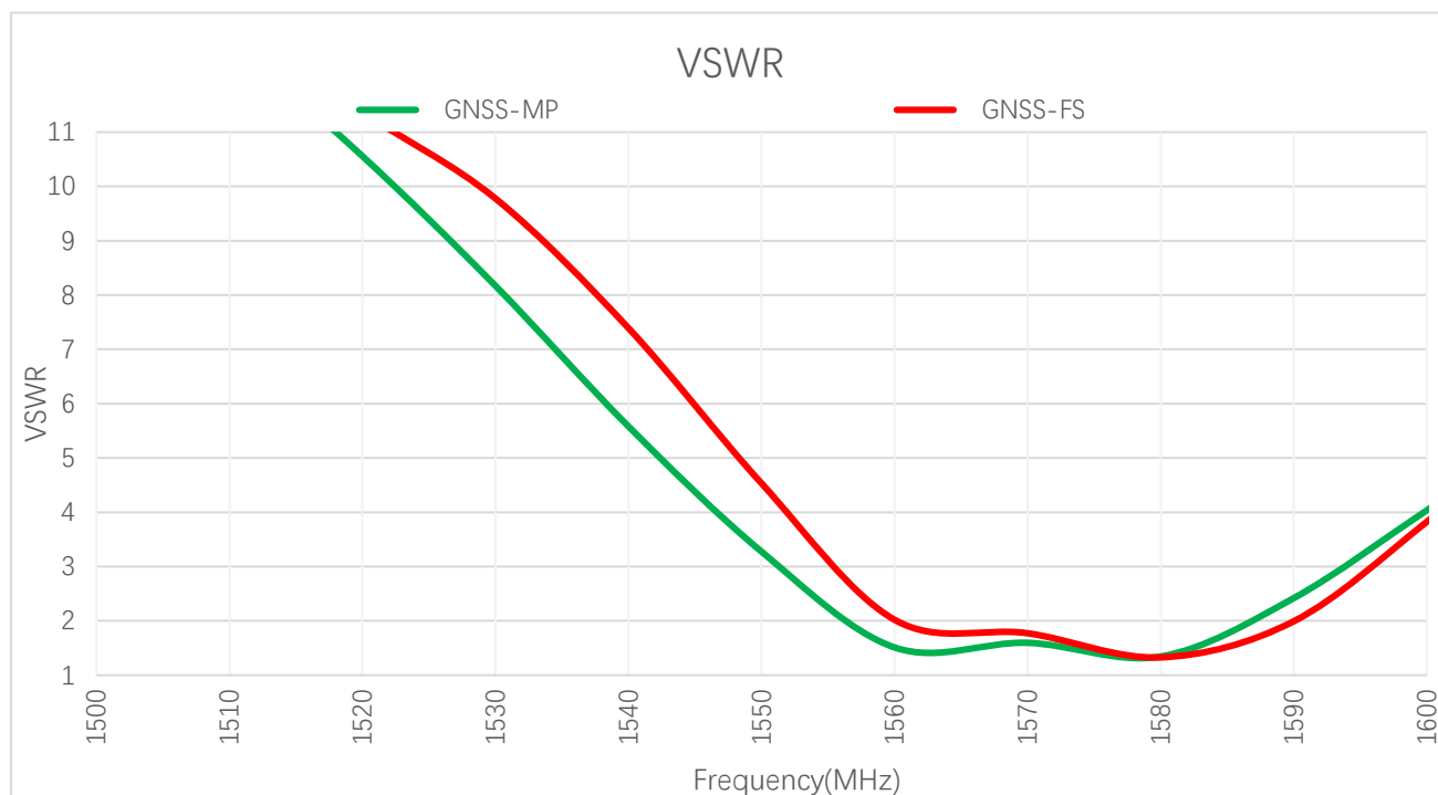
VSWR - GNSS
