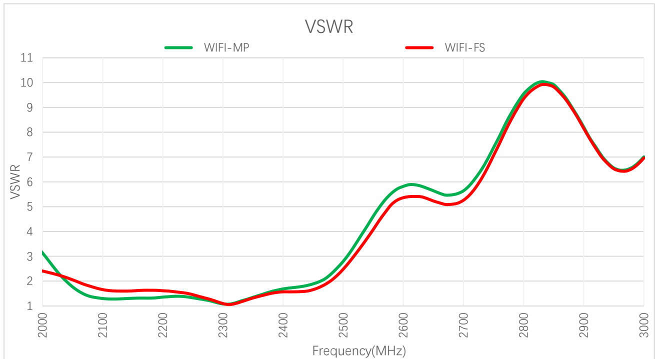
VSWR - Wi-Fi
