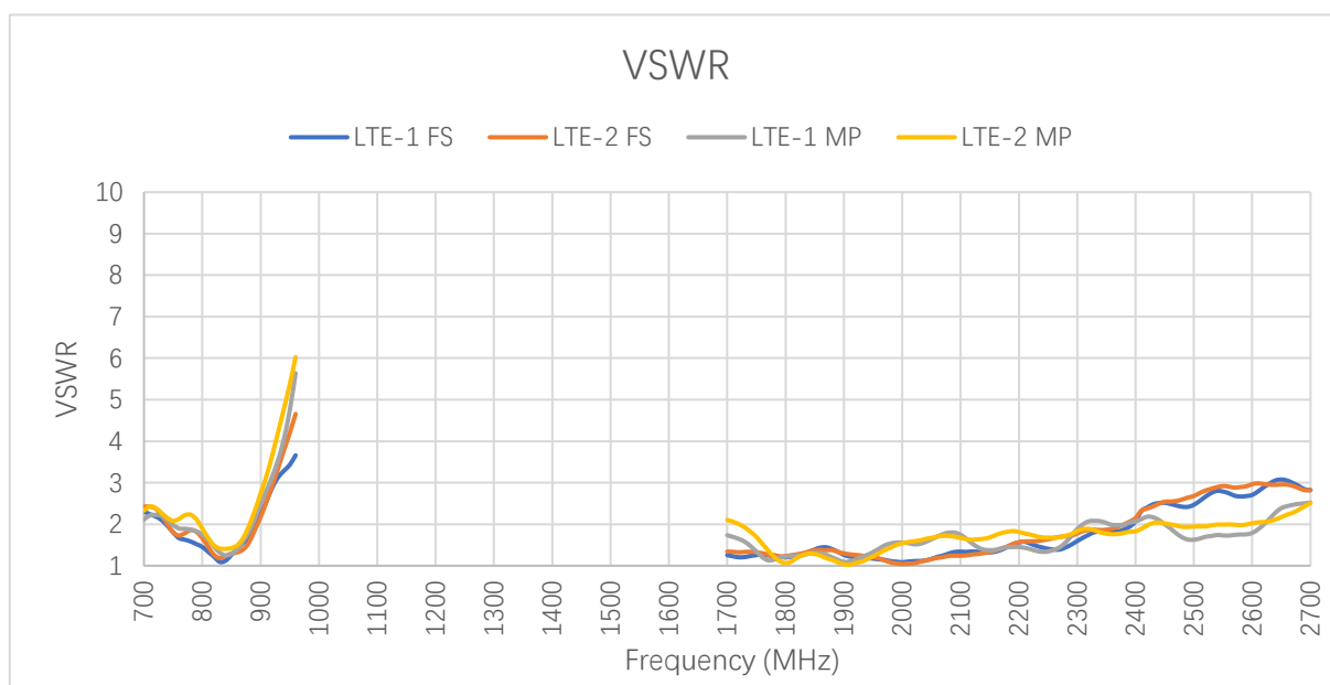
VSWR - LTE
