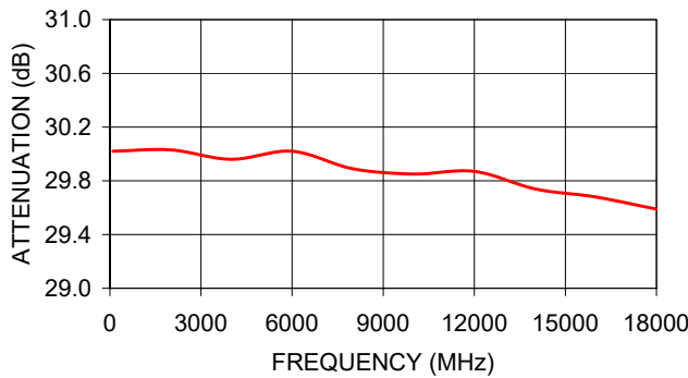
BW-S30W5+ ATTENUATION
