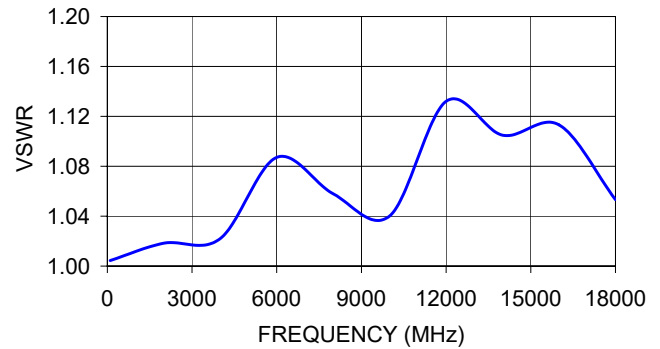
BW-S30W5+ VSWR
