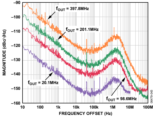
图16. 残留相位噪声, 1 GHz工作频率, 50 MHz参考时钟频率, 20x PLL乘法器
