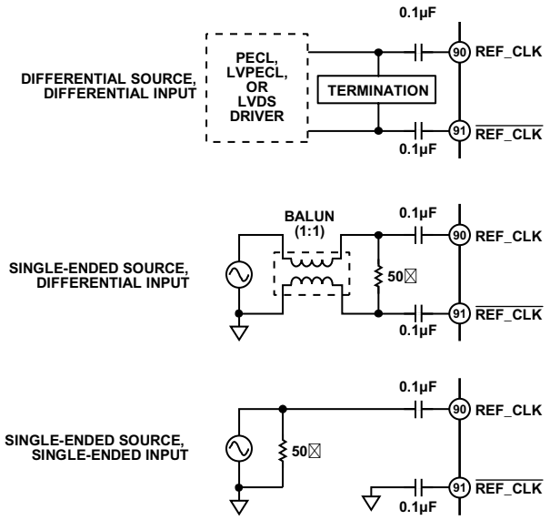
图32. 直接连接图
