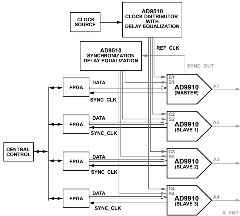
图20. 用AD9910作为参考和同步时钟分配器同步多个器件可以增大通道容量
